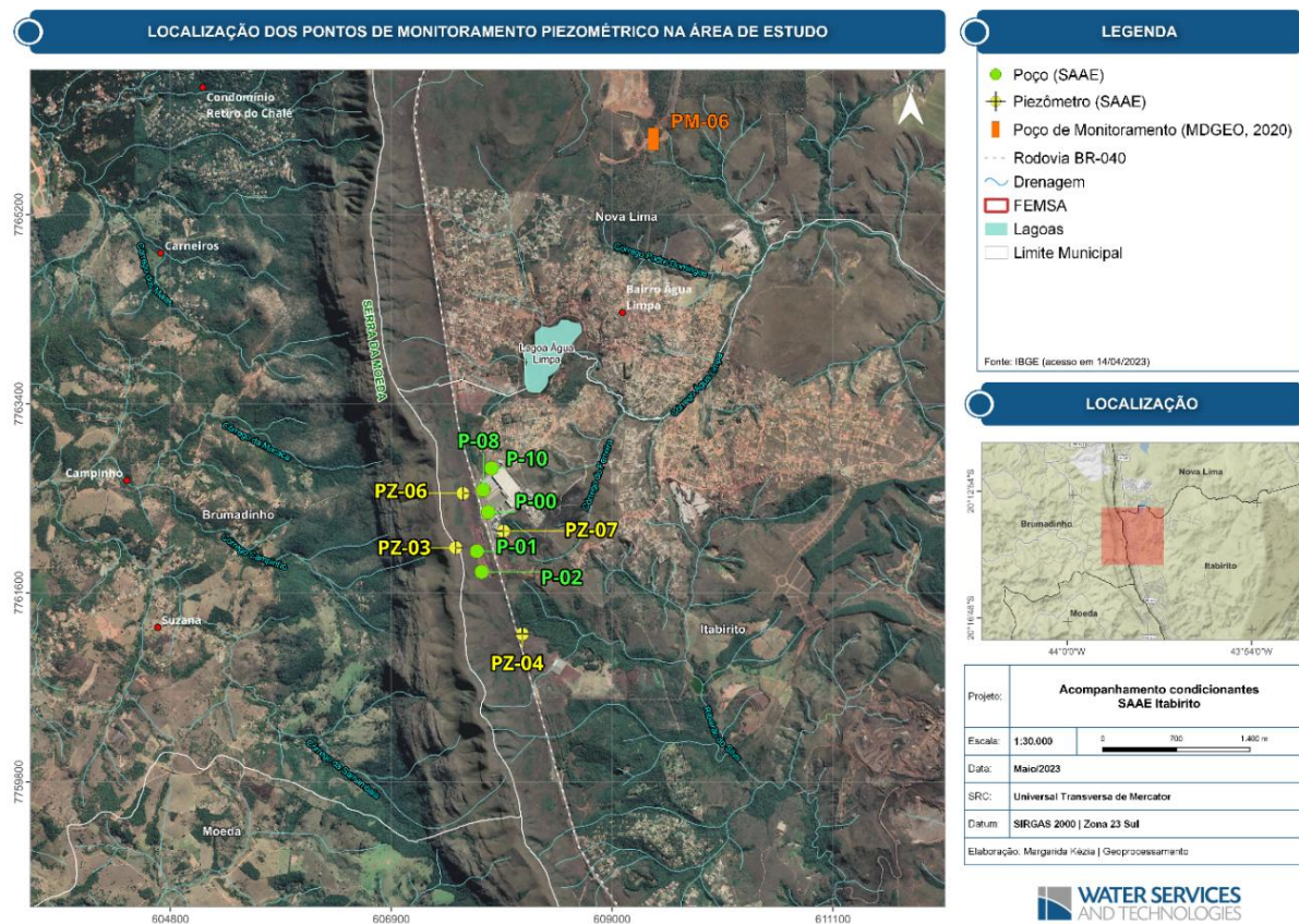
Figura 3-11: Distribuição espacial dos pontos de monitoramento do nível d'água subterrâneo.
