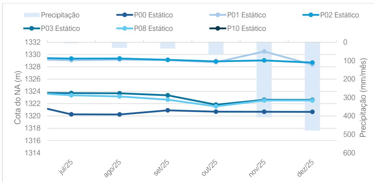
Figura 3-15: Variação da cota de nível d'água dos poços ao longo do segundo semestre de 2025.
