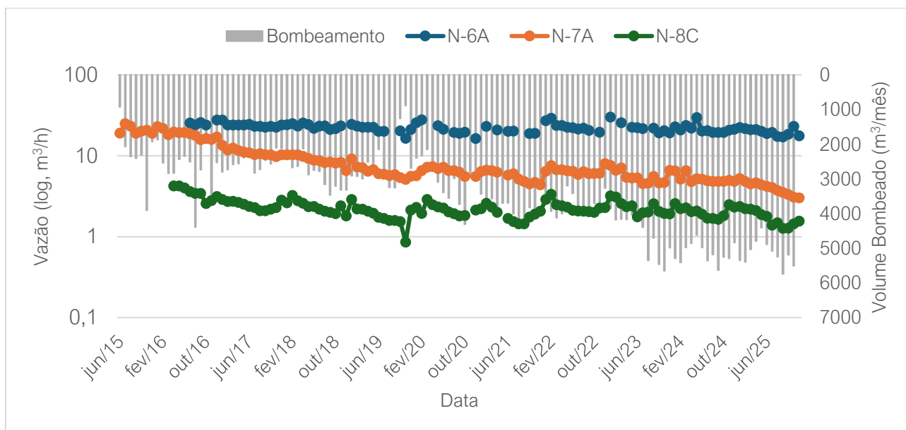
Figura 3-25: Vazão monitorada para os pontos N-6A, N-7A e N-8C, em função volume total bombeado pelos poços de abastecimento.
