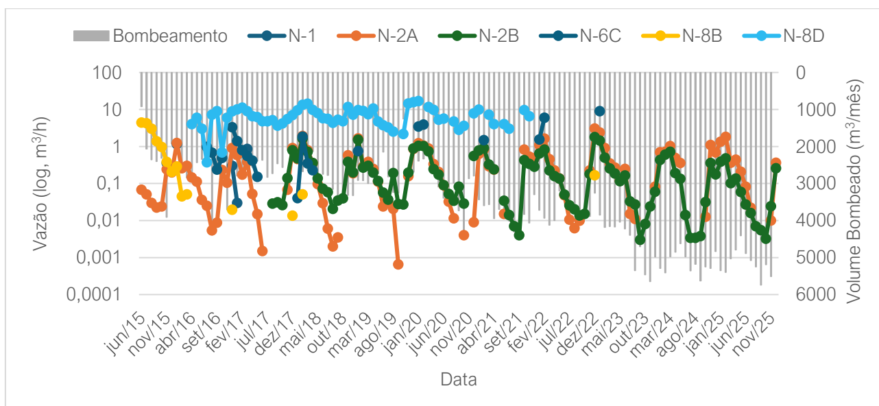
Figura 3-19: Vazão monitorada para os pontos N1; N-2A; N2-B; N-6C; N-8D e N8B, em função volume total bombeado pelos poços de abastecimento
