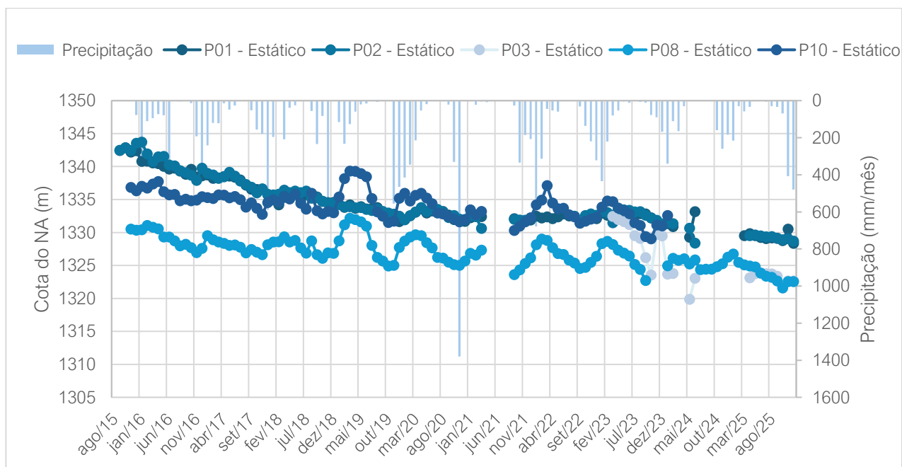
Figura 3-12: Monitoramento do nível d'água subterrâneo nos poços P01, P02, P08, P10 e P03 em função da precipitação mensal.
