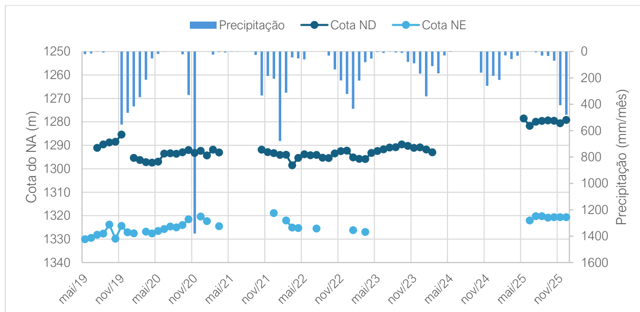
Figura 3-13: Monitoramento do nível d'água subterrâneo no poço P00 em função da precipitação mensal.
