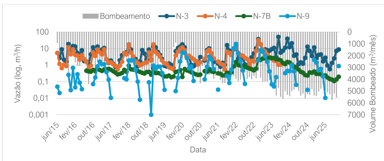
Figura 3-23: Vazão monitorada para os pontos N-3, N-4, N-7B e N-9, em função volume total bombeado pelos poços de abastecimento.
