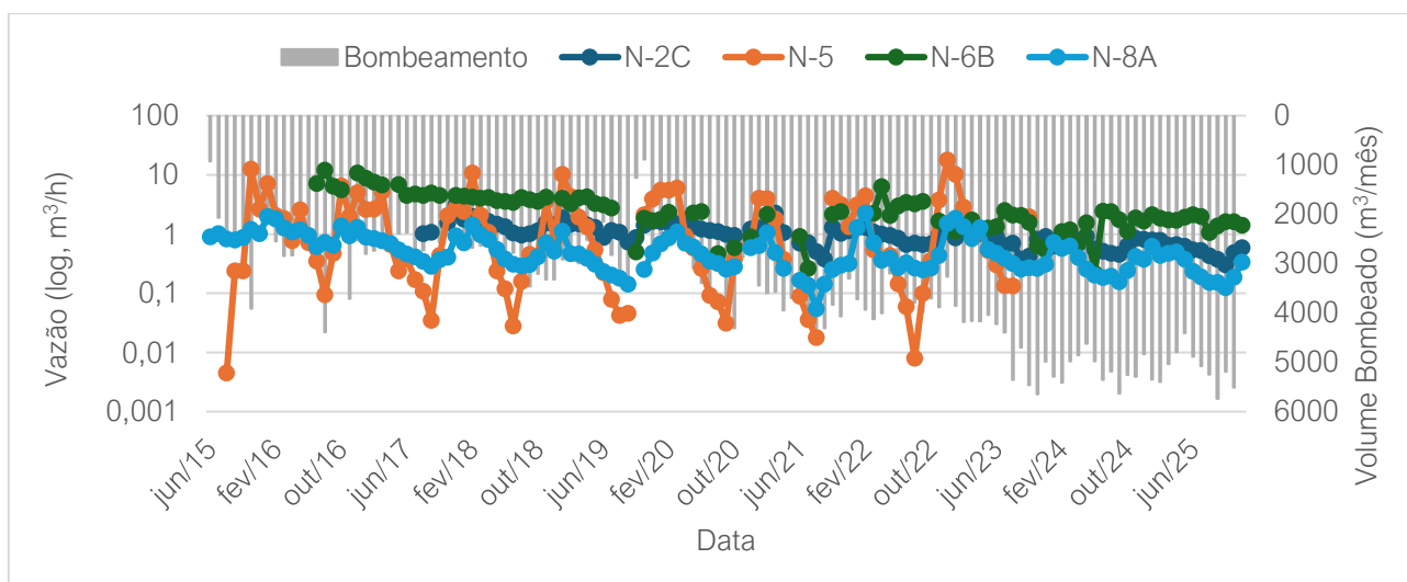
Figura 3-21: Vazão monitorada para os pontos N-2C, N-5, N-6B e N-8A, em função volume total bombeado pelos poços de abastecimento.
