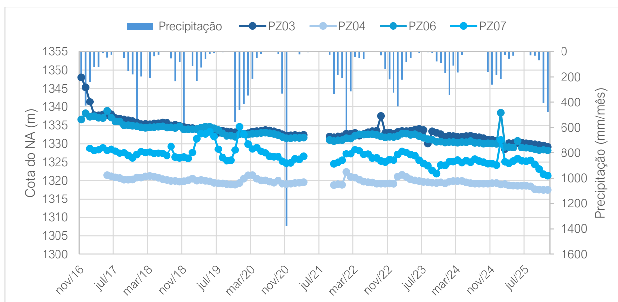
Figura 3-14: Monitoramento do nível d'água subterrâneo nos instrumentos PZ-03, PZ-04, PZ-06 e PZ-07, em função da precipitação mensal.
