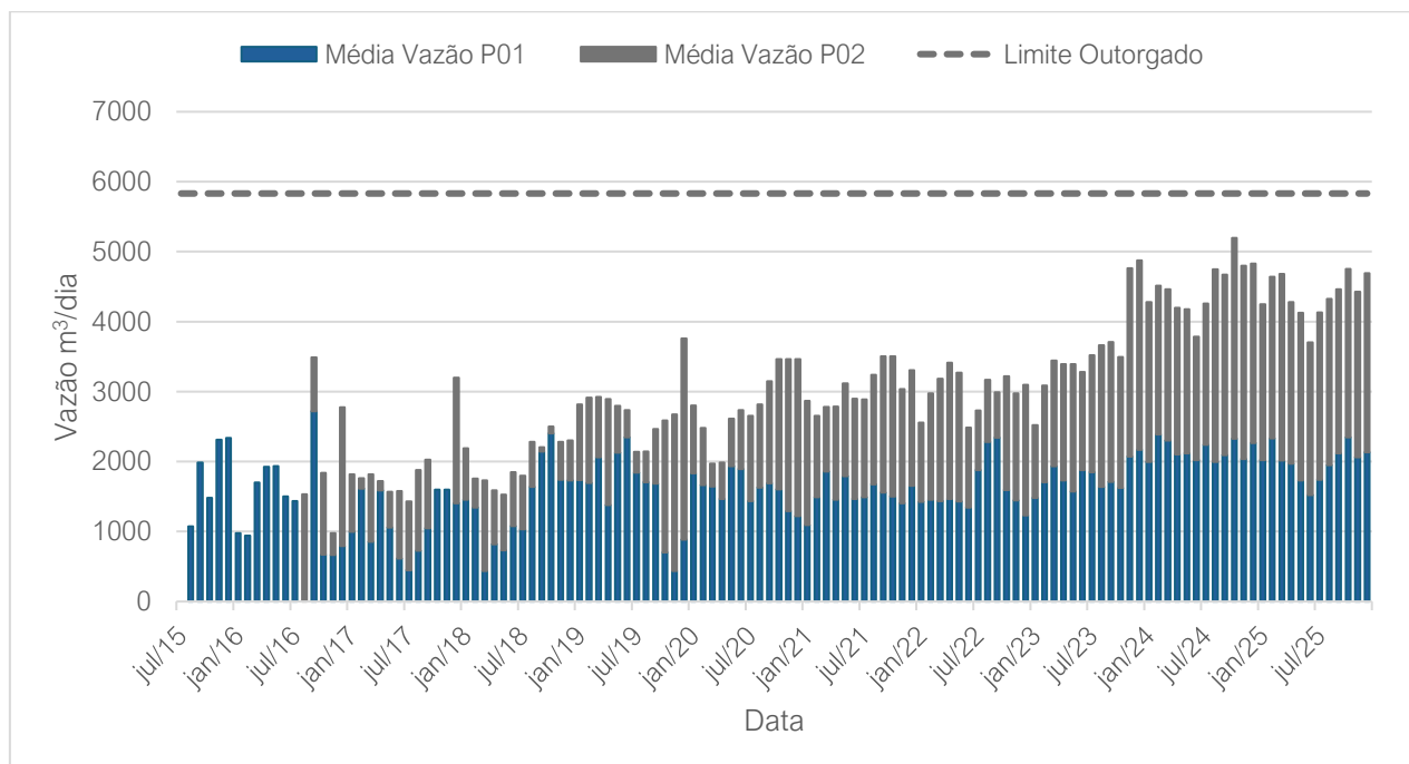
Figura 3-10: Vazão diária explorada em m³/d dos poços P01 e P02, e limite outorgado.
