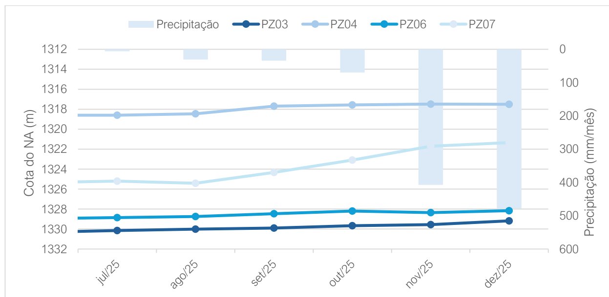
Figura 3-16: Variação das cotas de nível d'água dos piezômetros ao longo do segundo semestre de 2025
