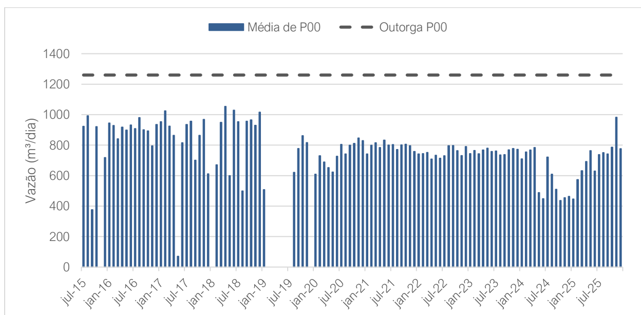
Figura 3-9: Vazão média mensal para o Poço P00, e limite outorgado.
