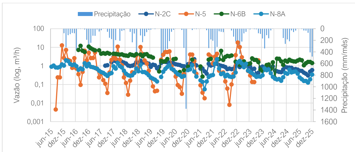
Figura 3-20: Vazão monitorada para os pontos N-2C, N-5, N-6B e N-8A, em função da precipitação.
