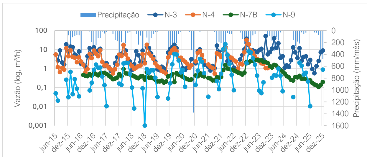
Figura 3-22: Vazão monitorada para os pontos N-3, N-4, N-7B e N-9, em função da precipitação
