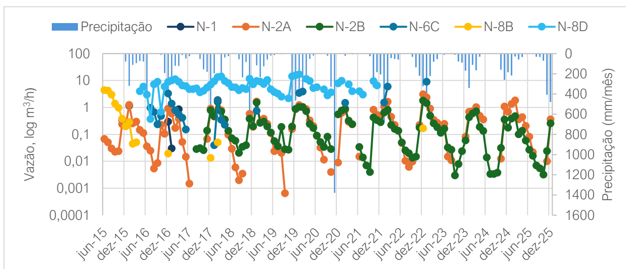
Figura 3-18: Vazão monitorada para os pontos N1; N-2A; N2-B; N-6C; N-8D e N8B, em função da precipitação.
