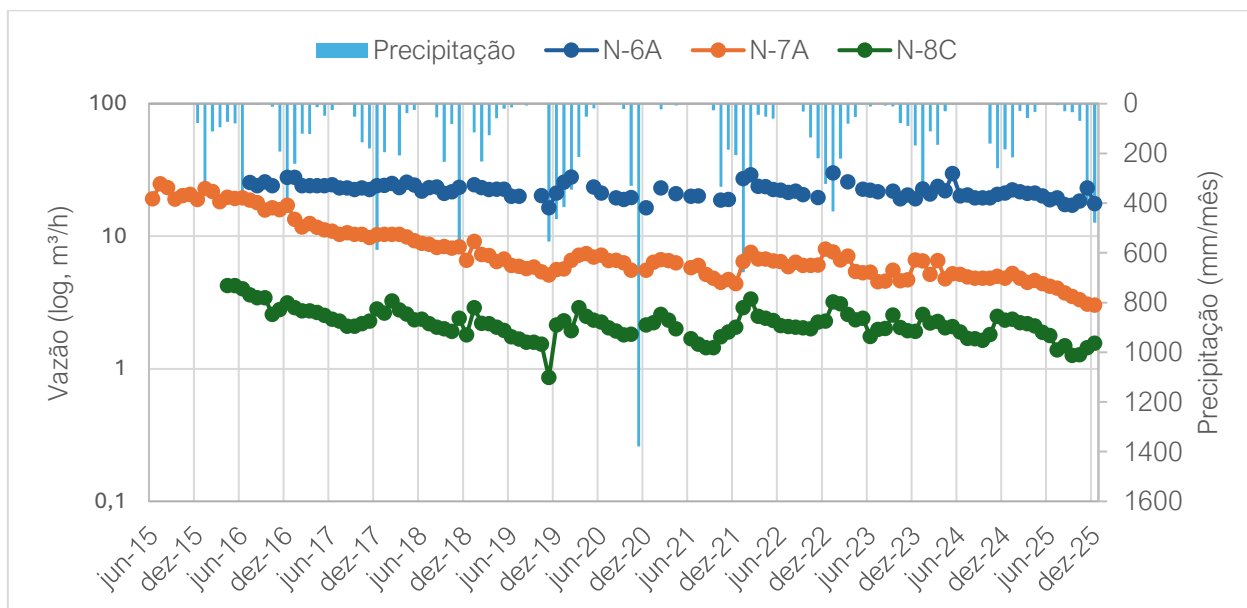
Figura 3-24: Vazão monitorada para os pontos N-6A, N-7A e N-8C, em função da precipitação.
